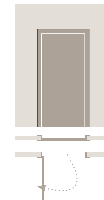
porta a battente hinged door porte à battant puerta batiente Flügeltür распашная дверь L 600/650/700/750/800/900 H 2000/2100
